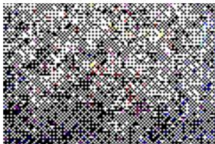
Dithering Zorganizowany
